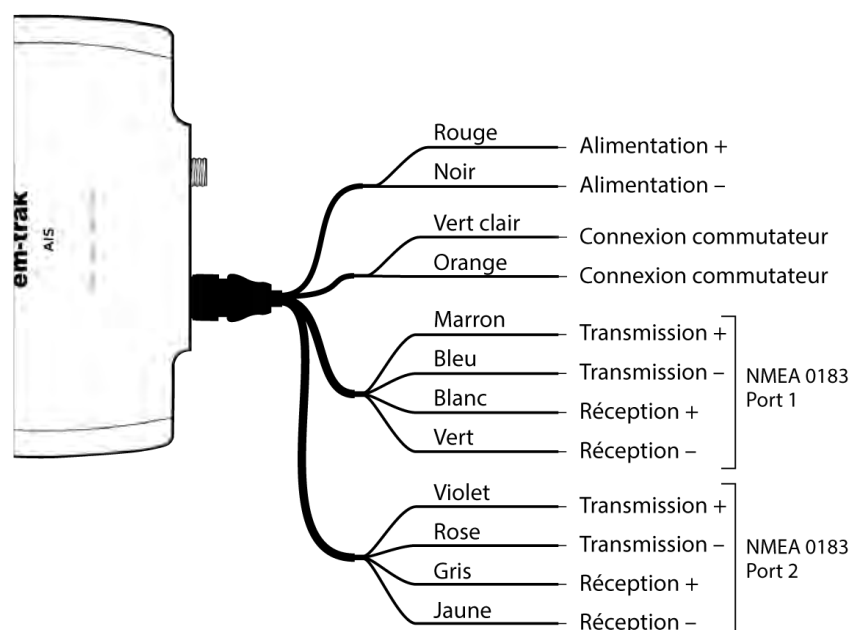
Illustration 9 : Connexions du câble d'alimentation et de données
