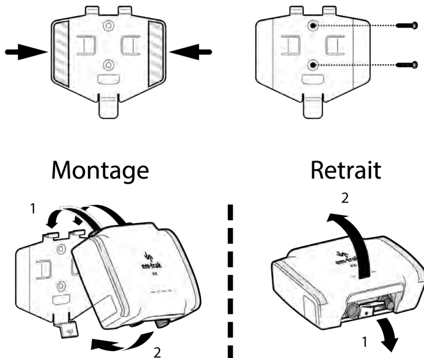
Illustration 13 : Émetteur-récepteur montage
