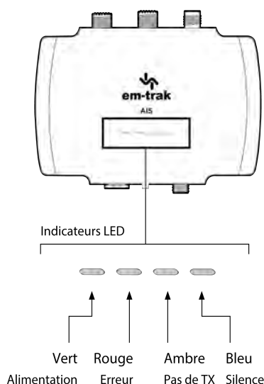
Illustration 21 : Emplacement des indicateurs LED sur l'unité émetteur-récepteur SIA
